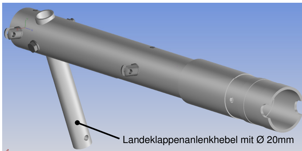
Bild 2 Landeklappenverteiler (links)
